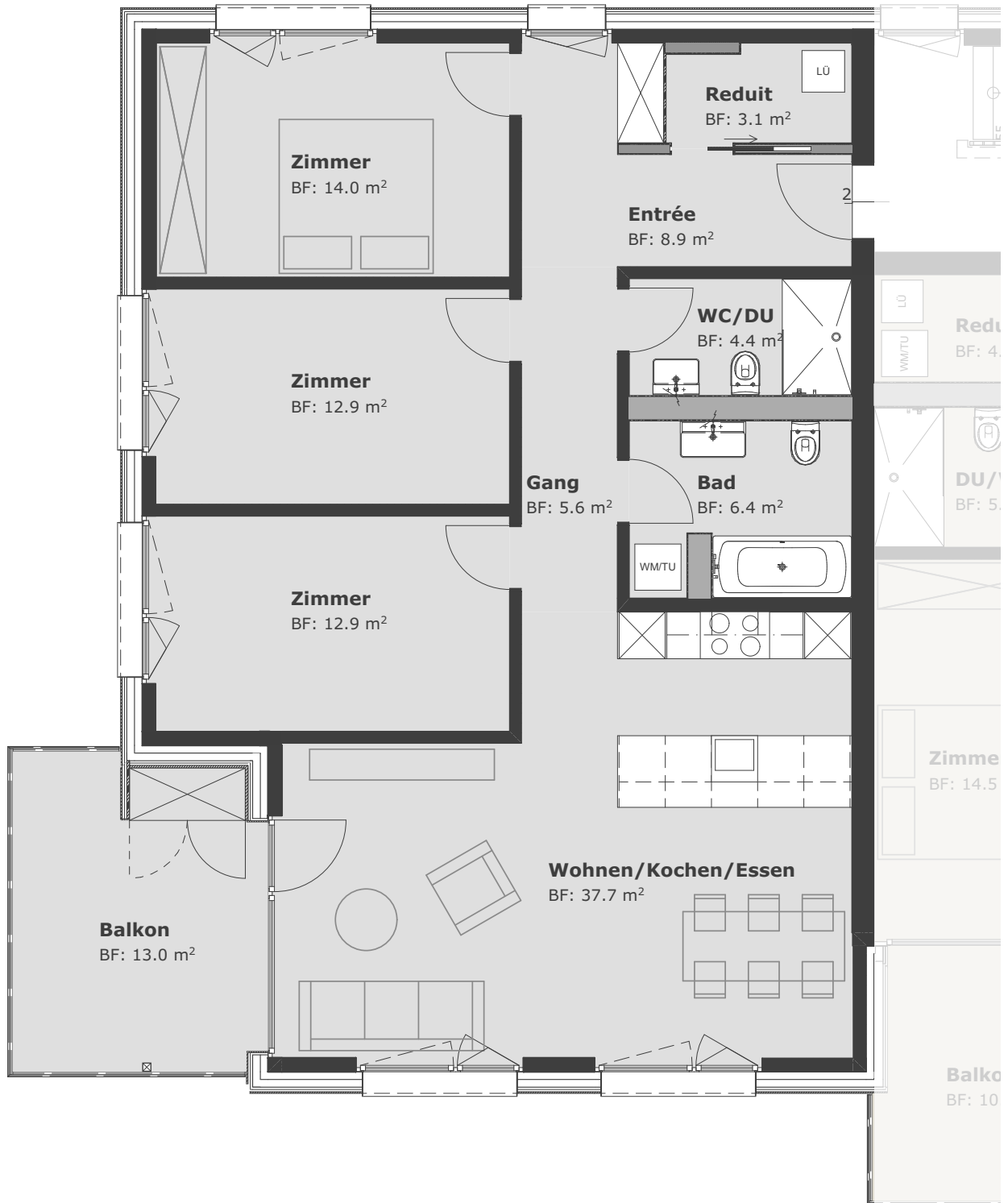
WOHNUNG B.3.1
